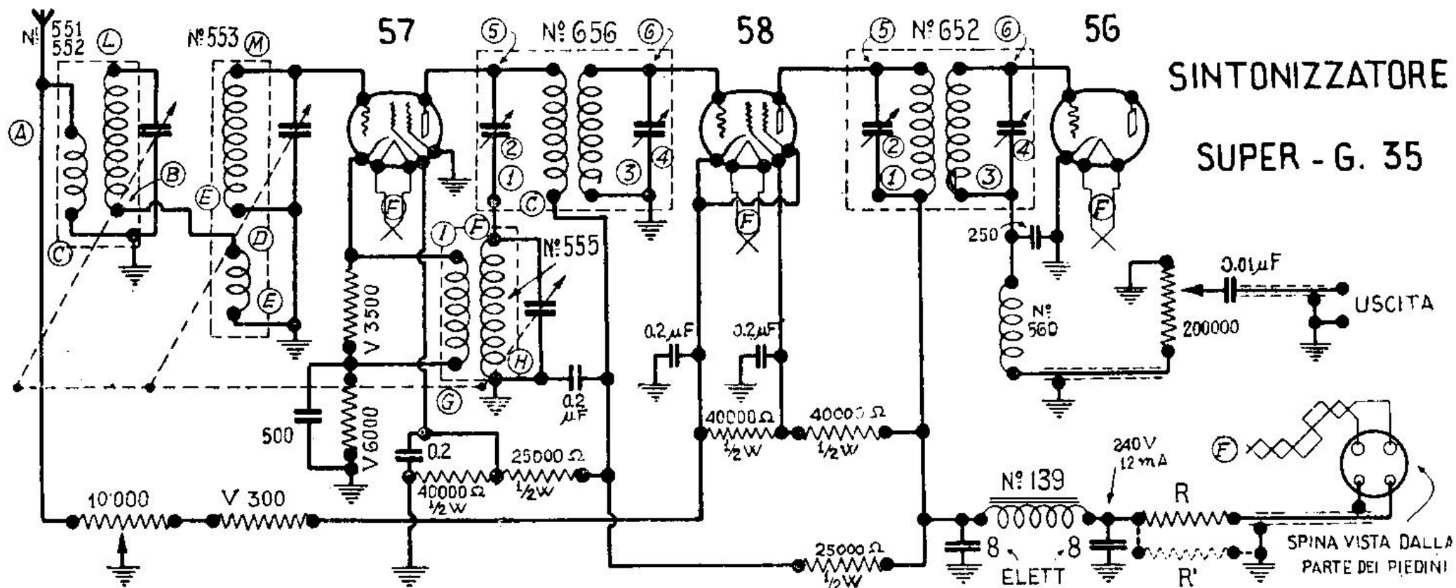
FIG. 2. - Lo schema elettrico del G-35.
